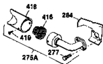
OPTIONAL SPARK ARREST MUFFLER
