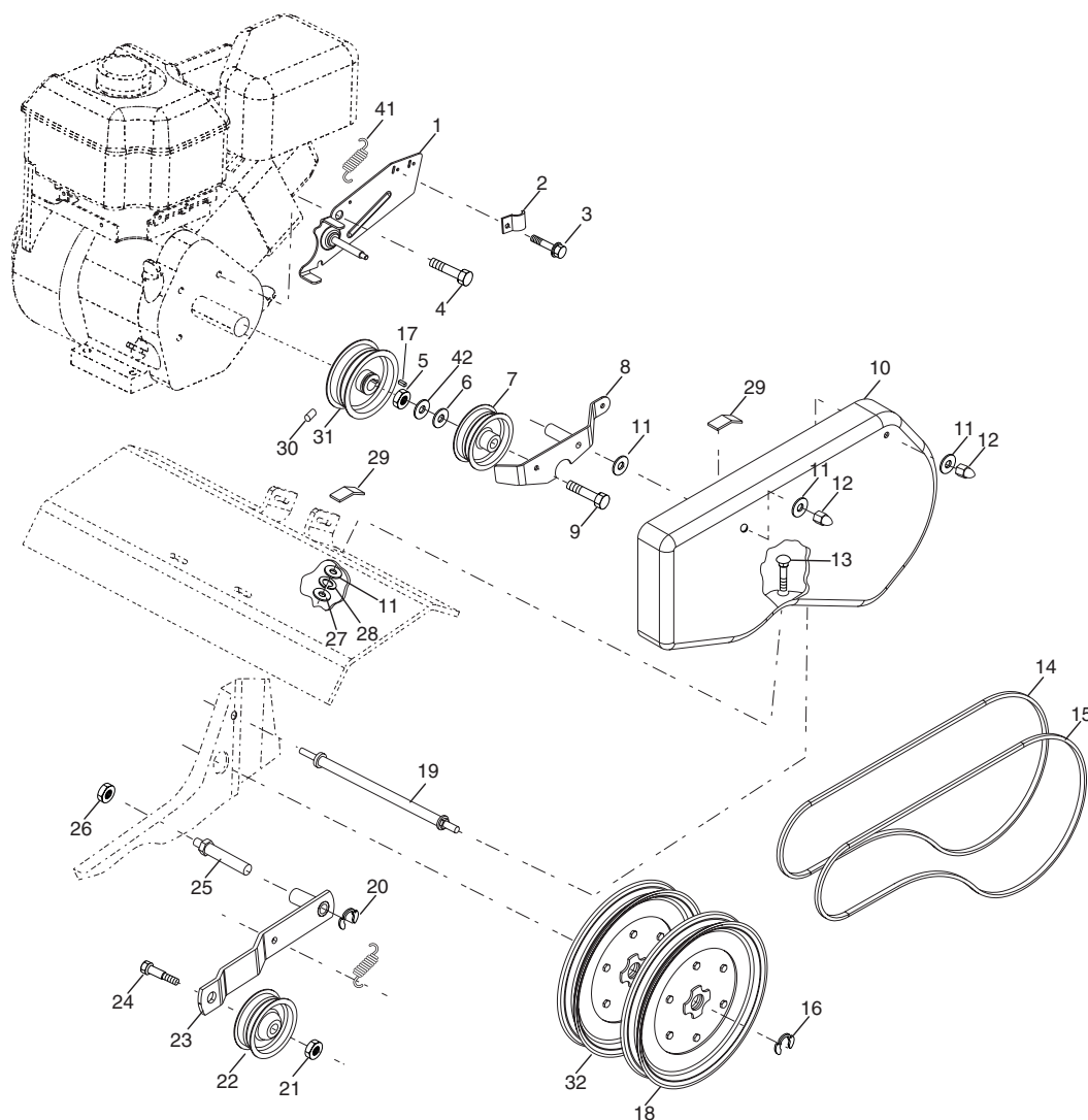
belt_guard_14
