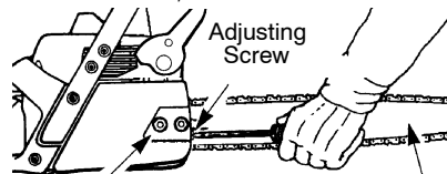
Guide Bar
