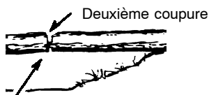
Première coupe du côté de compression du rondin
