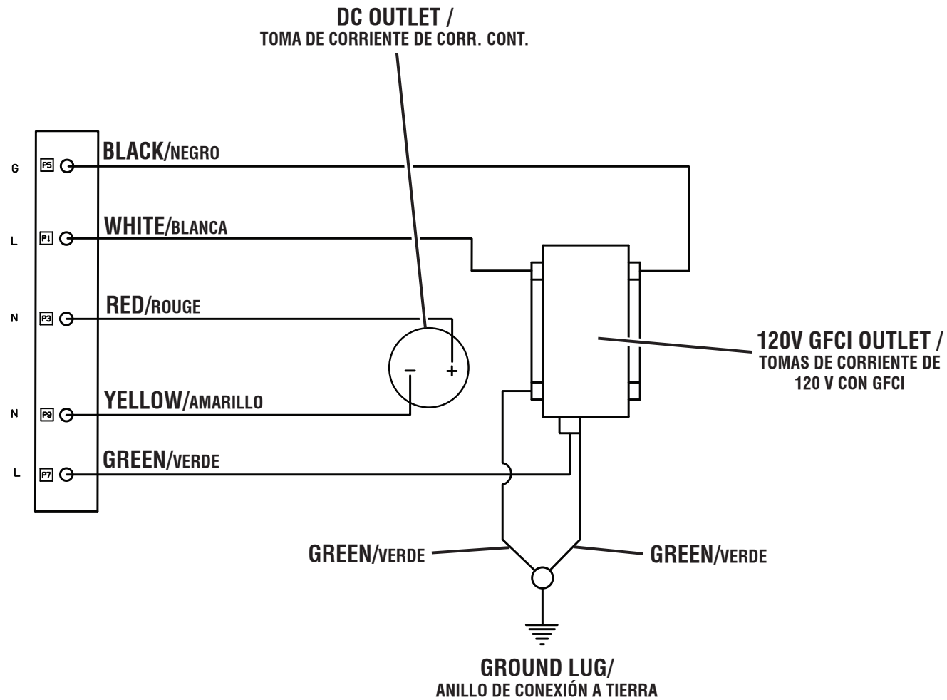
WIRING DIAGRAM / DIAGRAMA DE CABLEADO
