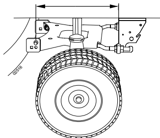
Los Varillajes Delanteros Deben Ser De Igual Longitud
