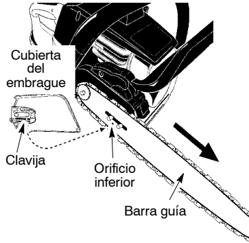
Vista interior de la cubierta del embrague
