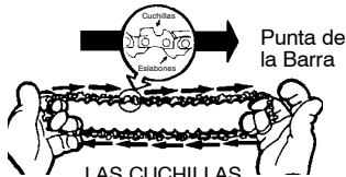
LAS CUCHILLAS DEBERÁN APUNTAR EN DIRECCION A LA ROTACION
