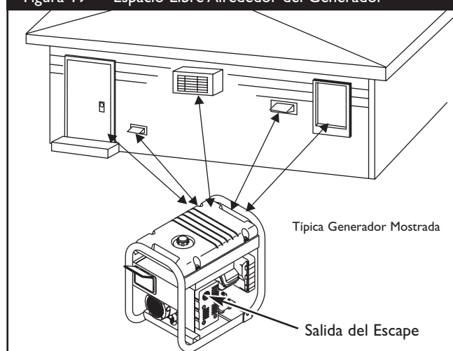
Figura 19 — Espacio Libre Alrededor del Generador
