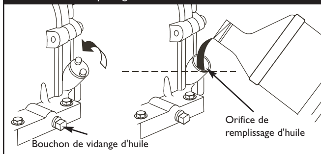
Figure 31 — Bouchon de vidange d'huile et bouchon de remplissage d'huile
