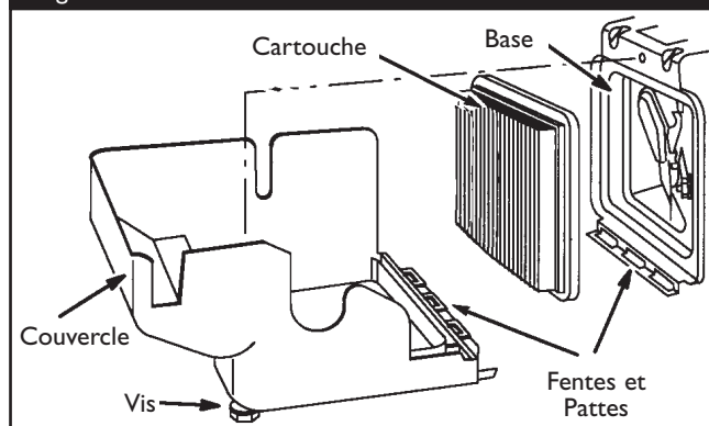
Figure 32 - Filtre à air
