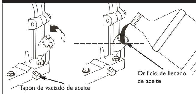
Figura 48 — Tapón de vaciado de aceite y tapón de llenado de aceite
