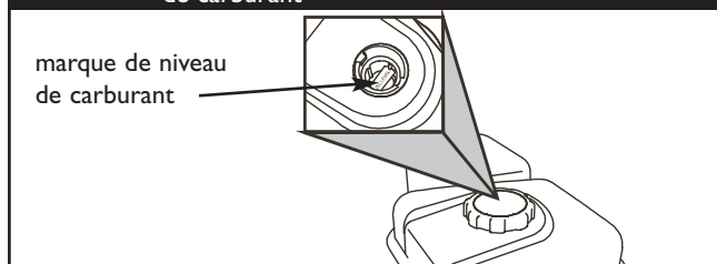
Figure 18 - Ajouter de l'essence jusqu'à la marque de niveau de carburant
