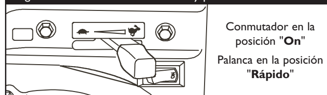
Figura 44 — Conmutador ON/OFF y palanca de velocidad
