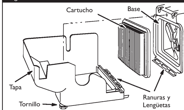
Figura 49 - Filtro de aire
