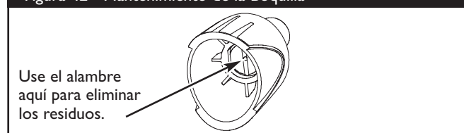
Figura 42 - Mantenimiento de la Boquilla
