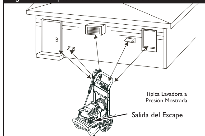
Figura 29 — Espacio Libre Alrededor del Lavadora a Presión
