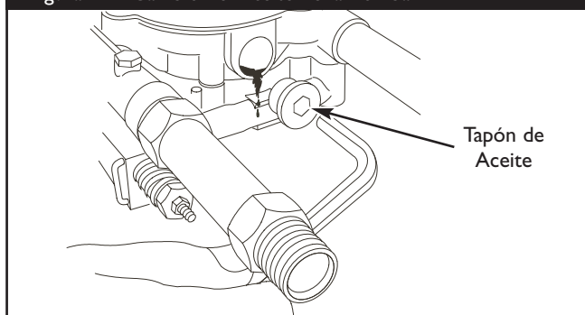
Figura 44 - Cambio del Aceite de la Bomba
