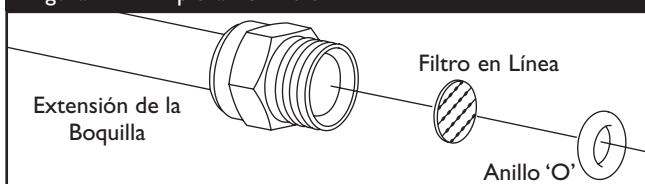
Figura 41 - Limpieza del Filtro
